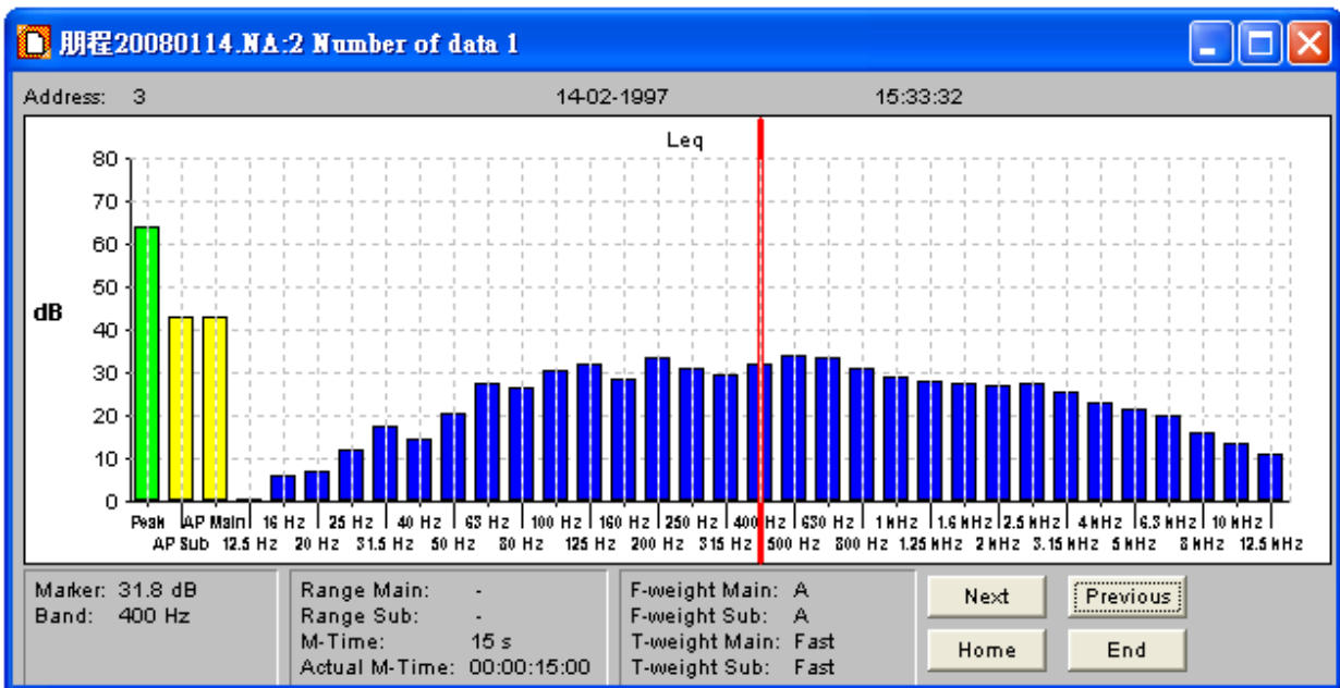
背景音頻譜柱狀圖
