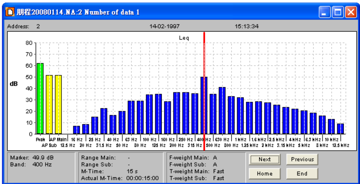
施工前噪音頻譜柱狀圖
