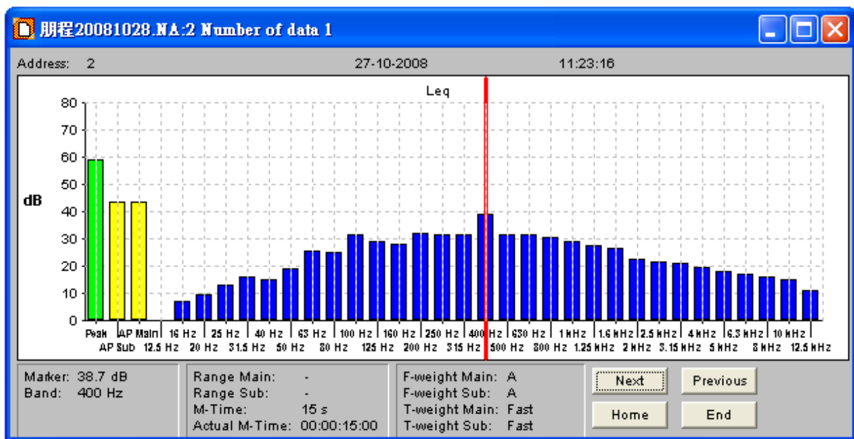
施工後噪音頻譜柱狀圖
